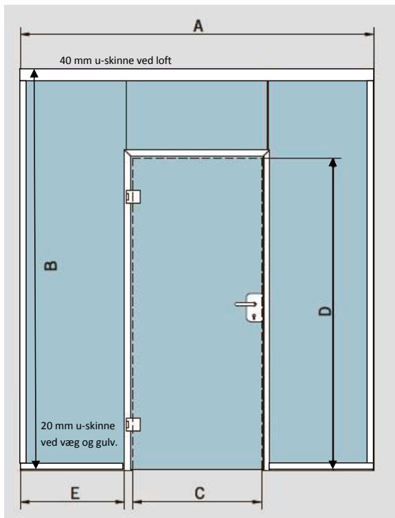
U-profil 20x20x20 til gulv og væg
