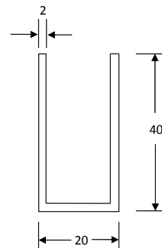
U-profil 40x20x40 til loft
