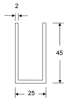
U-profil 45x25x45x2 til loft
