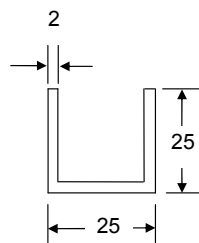
U-profil 25x25x25x2 til gulv og væg
